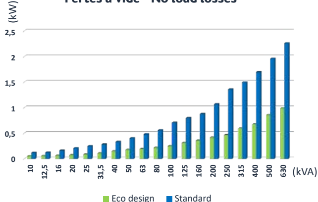
Pertes à vide - No load losses
